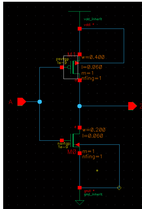
Esquemático no nível de transistores
