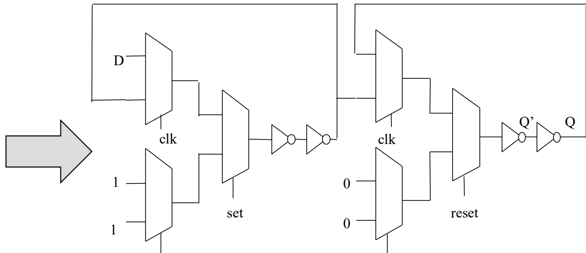
Implementação de FLIP-FLOP MESTRE-ESCRAVO com SET e RESET
